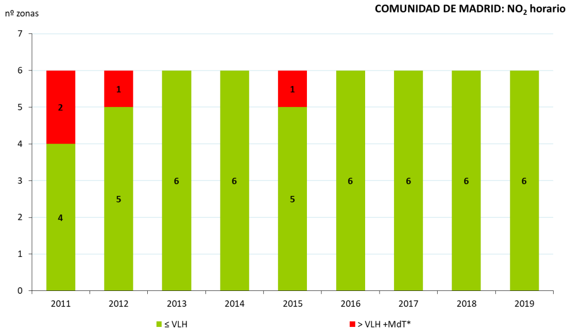
Figura 153. Situación respecto al VLH de NO 2 (2011-2019)
