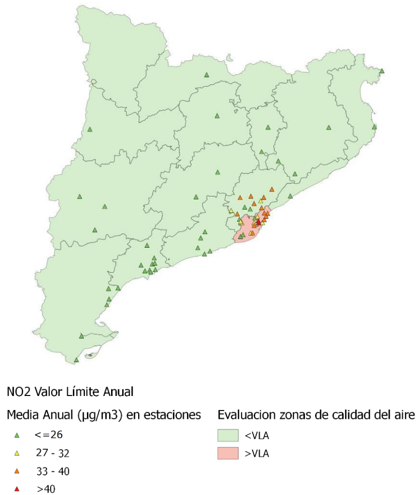
Figura 111. Media anual en estaciones y evaluación por zonas del VLA de NO 2
