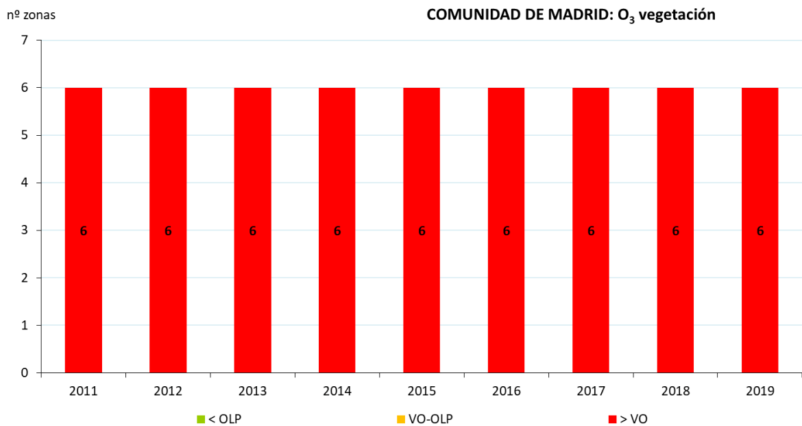
Figura 156. Situación respecto al VO-Vegetación de O 3 (2011-2019)
