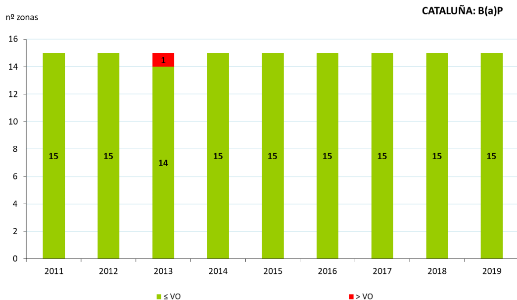
Figura 121. Situación respecto al VO de B(a)P (2011-2019)
