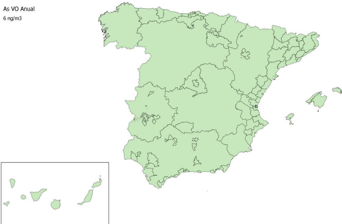
Figura 29. Situación de la calidad del aire de 2019 respecto del VO de As
