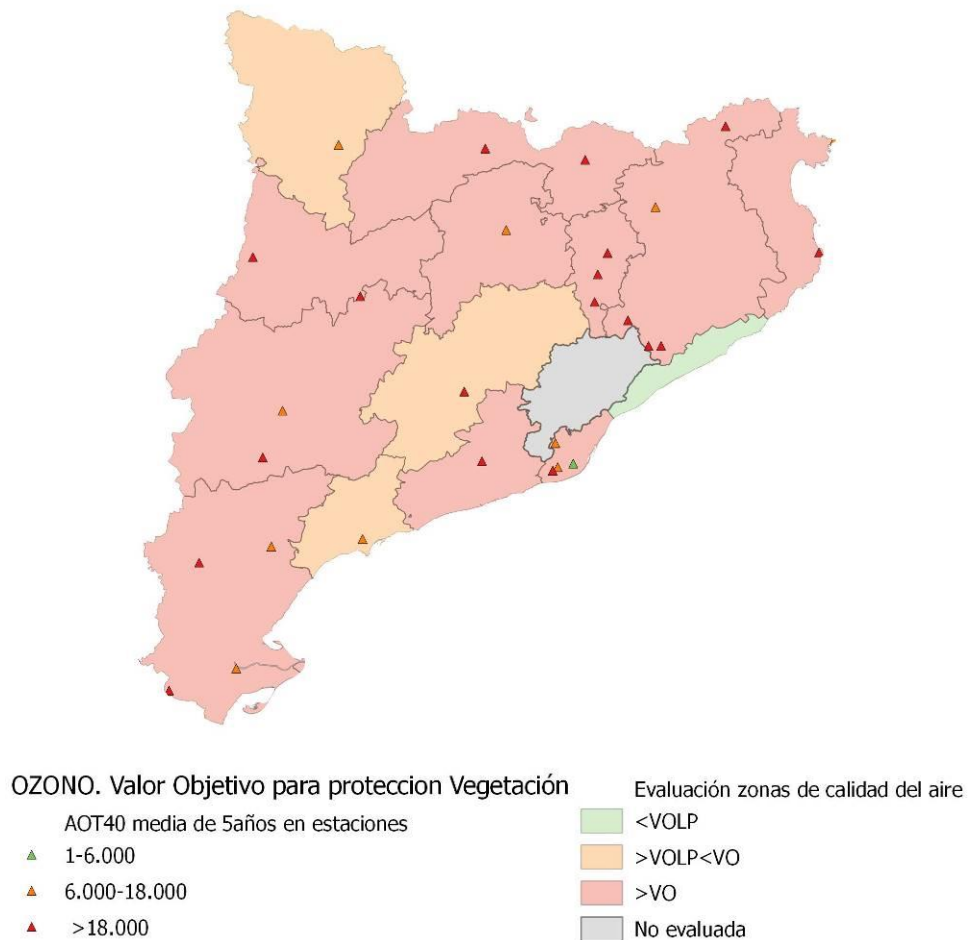
Figura 115. Número de superaciones en estaciones y evaluación por zonas del VO de O 3 para la protección de la vegetación
